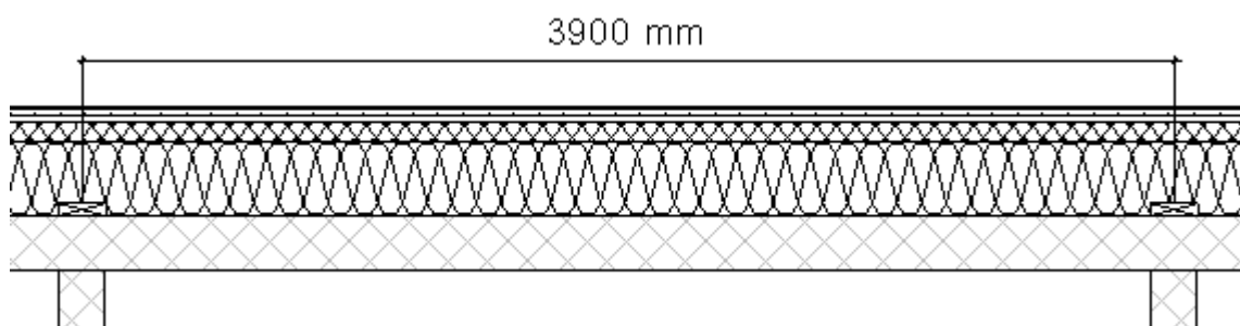
Figur 6.3: Bjälklagssektion för terrass.
