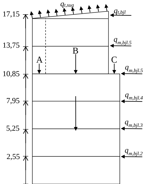
Figur N.1: Beräkningsmodell av stjälpande byggnad.
