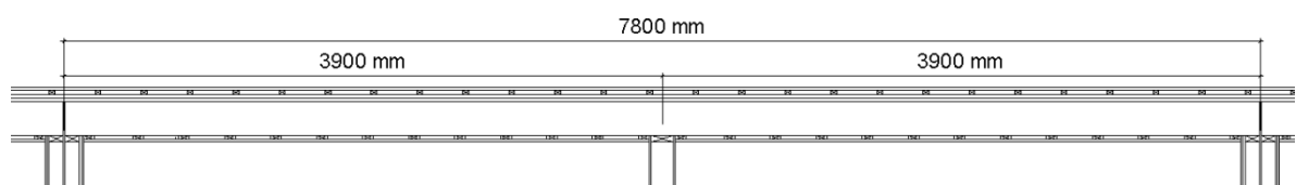
Figur 6.1: Takbalk upplagd på träregelväggar.
