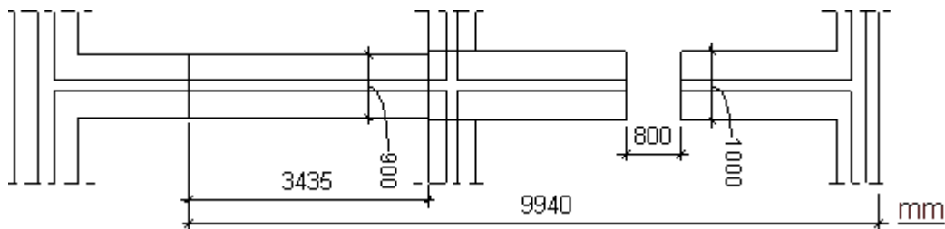
Figur N.3: Medverkande area för grundsula.
