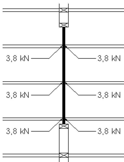
Figur 6.4: Avväxling i bjälklag, horizontalsnitt.
