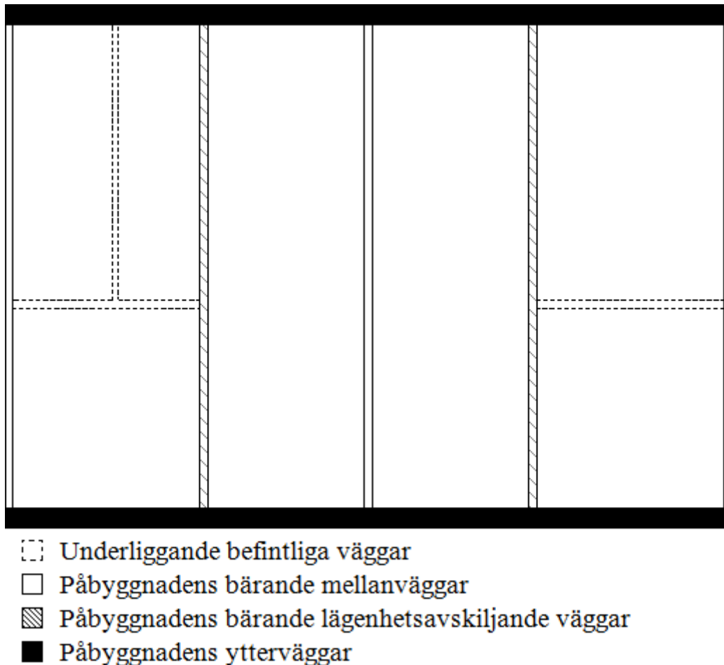
Figur 4.2: Snitt ur plan för påbyggnad.
