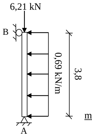
Figur J.6: Lastfall för en regel i yttervägg, vindlast – huvudlast.
