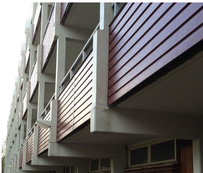
Figur 3.7: Sprickbildning i konsolbalkar (Fotograf: R. Friberg).
