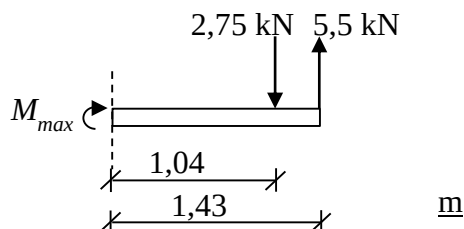
Figur G.6: Snitt i x_{max} – Fall 2.
