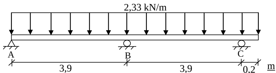
Figur J.7: Lastfall för balk vid en yttervägg, snölast – huvudlast.
