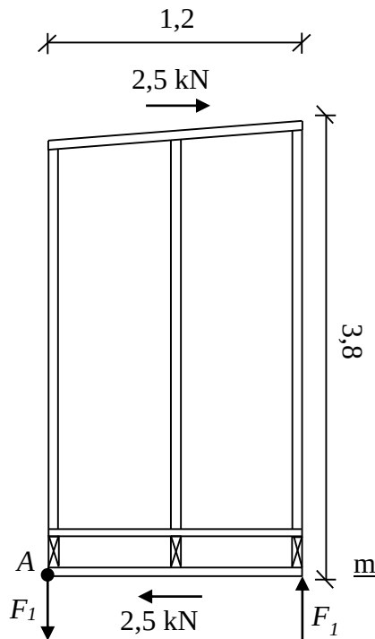
Figur J.2: Verkande krafter i mellanvägg på grund av vindlast.
