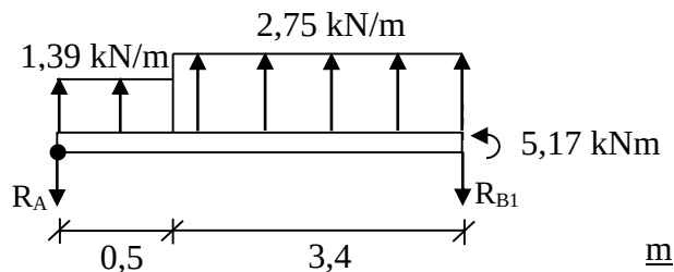
Figur H.5: Balkdel A-B – momentjämvikt.
