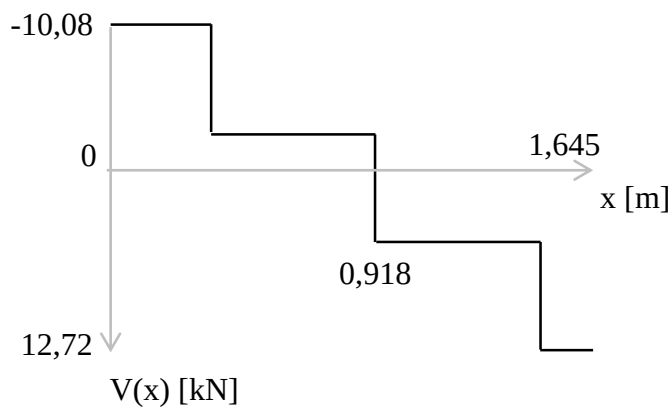
Figur I.3: Tvärkraftsdiagram.
