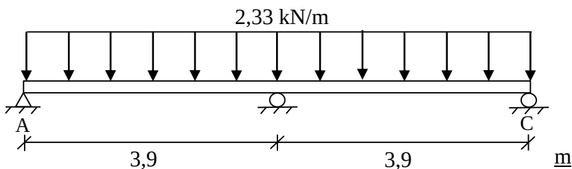
Figur H.1: Lastfall för takbalk.
