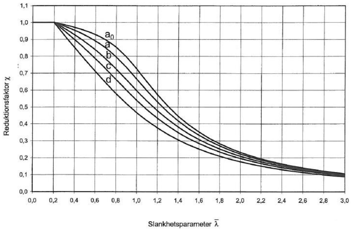
Figur 3.7 [i] – Reduktionsfaktorn \chi för olika knäckningskurvor och slankhetsparametrar.
