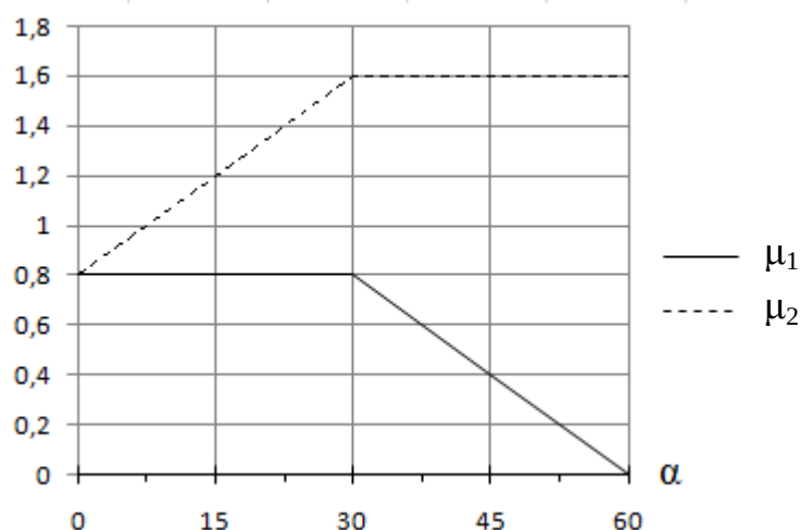
Figur 2.5 – Formfaktorer för pulpet- och sadeltak.
