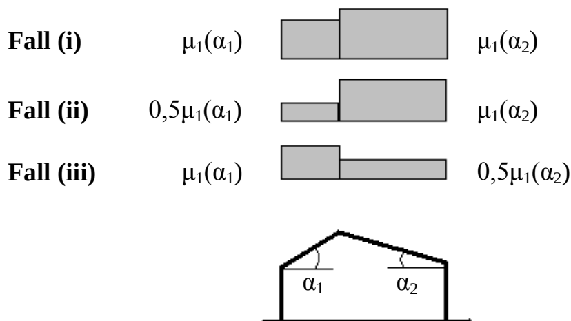
Figur 2.7 – Lastbild för snölast på sadeltak.
