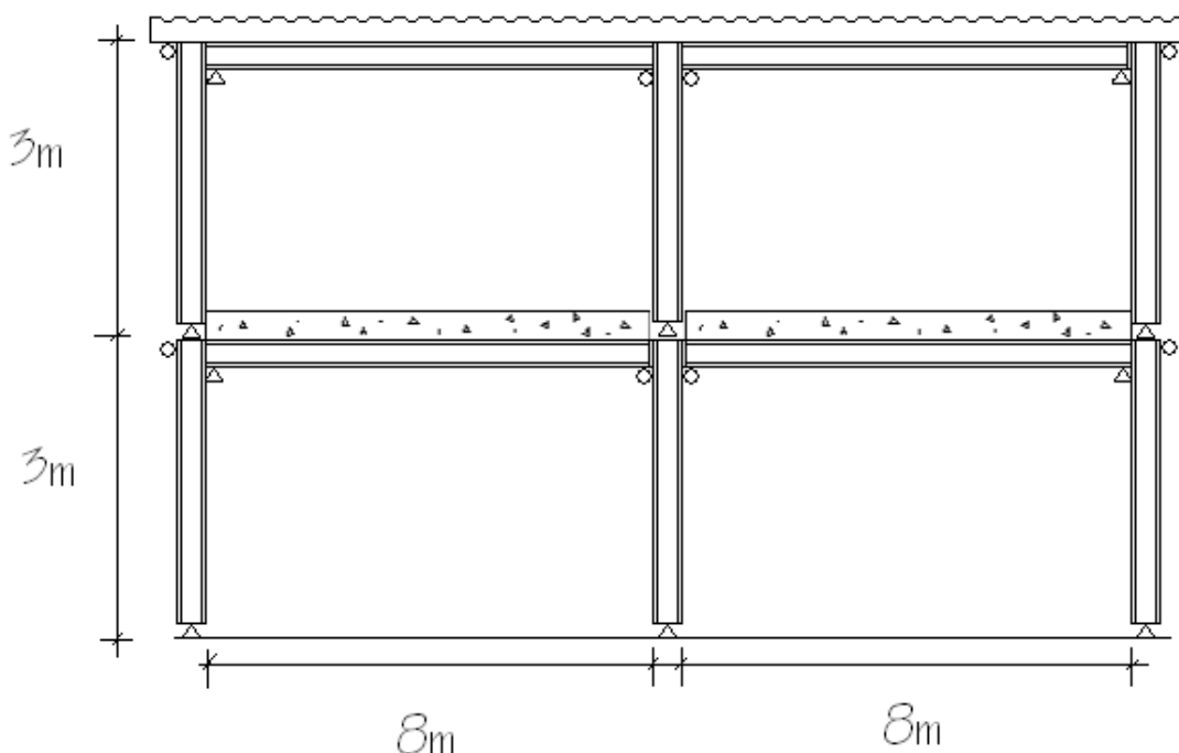
Figur 4.1 – Stomsektion.
