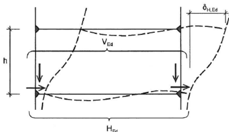
Figur 3.1 lml – Beteckningar för (3.3).
